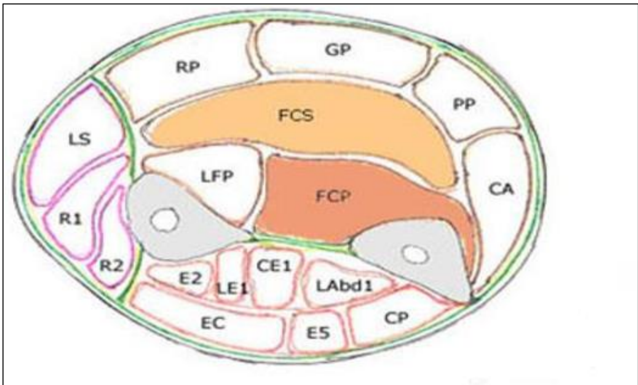
Coupe transversale au niveau du 1 /3 moyen de l'avant-bras
